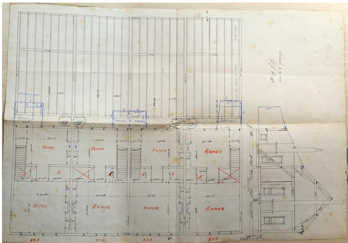
Afb. 14 Bouwtekening voor vier huisjes
